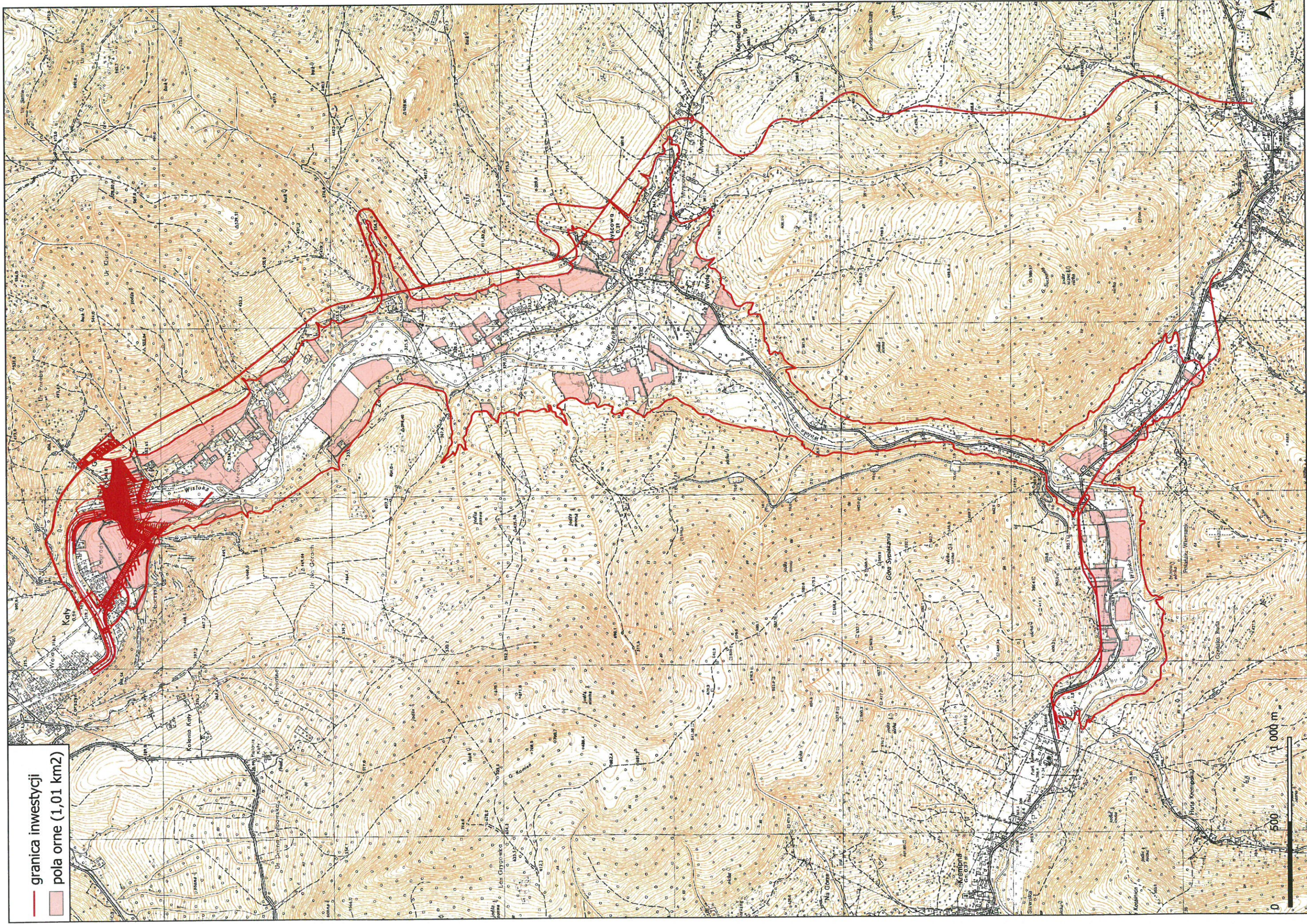
Zbiornik Kąty - Myscowa. Granica inwestycji Skala 1:20000
